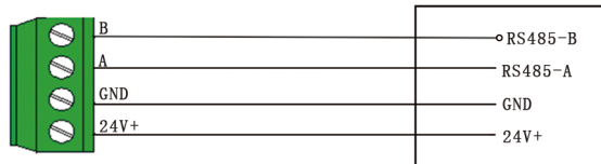
485输出型
