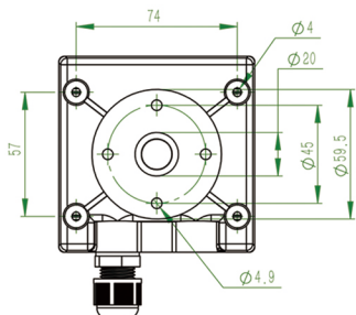
背面 (管道型)
