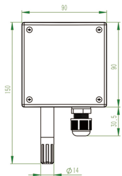
正面 (墙面型)
